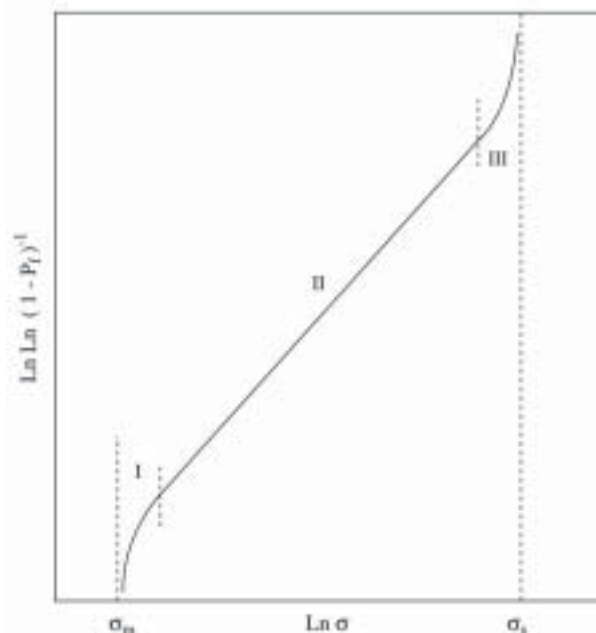
Figura 1. Diagrama de Weibull 3 .
